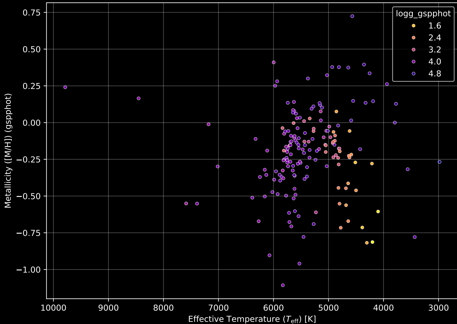
APOGEE DR17 Field: [047-41_MGA] Stellar Population Parameters (n= 174)
